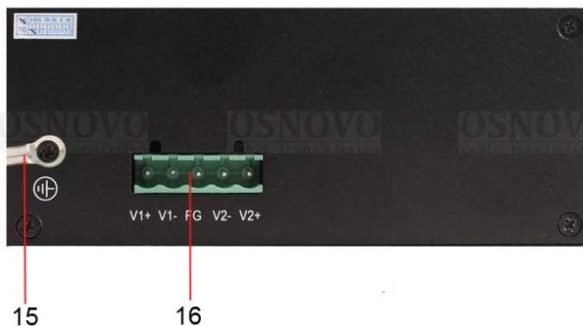
Рис. 3 Разъемы и индикаторы коммутатора SW-8082/IC
