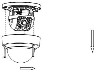
Рисунок 2-5 Демонтаж купола
